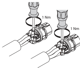
Kuva 14: Kiristä kotelo ruuvit
