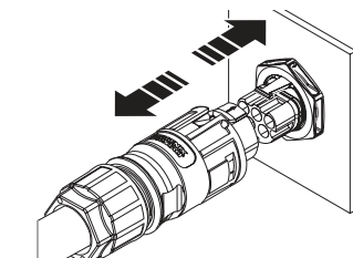
Kuva 30: Erota AC-liitinrunko
