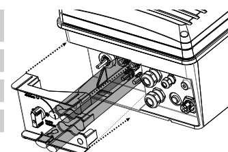
Kuva 26: Sulje liitinkansi
