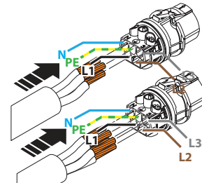
Kuva 13: Vaihda liitinrunko
