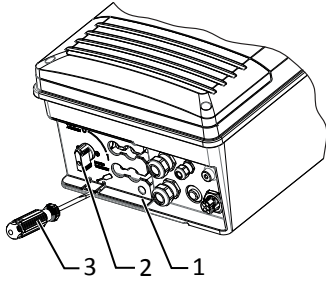
Kuva 9: Paljasta DC-liitântäalue
