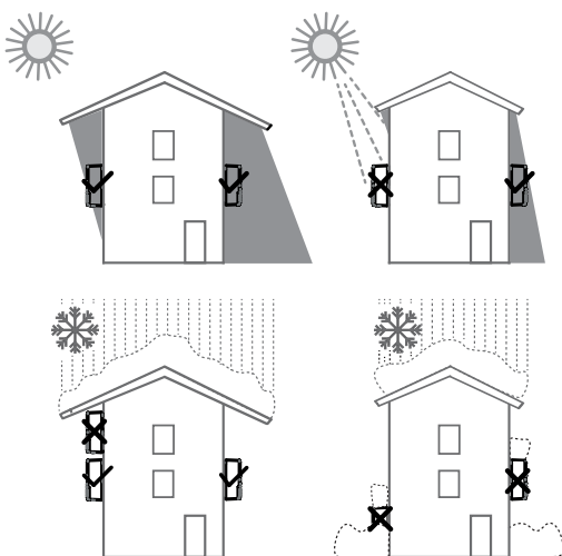
Kuva 3: Laite ulkoasennuksessa
