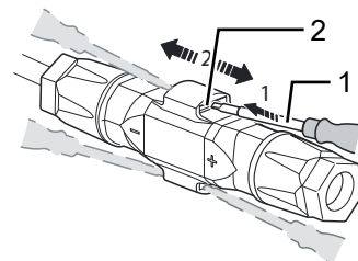
Kuva 32: Irrota liitin
