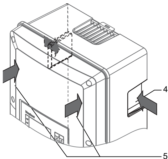
Kuva 6: Nosta laite ylös
