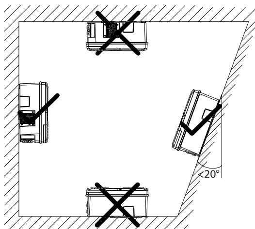
Kuva 4: Sallittu asennuspaikka
