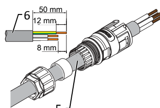
Kuva 12: Poista johdon eristys
