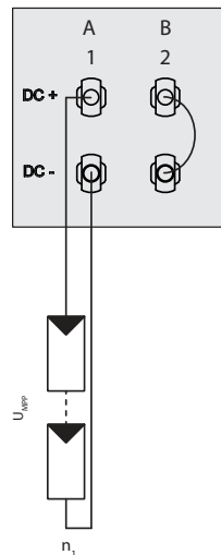
Kuva 22: Rinnakkainen tulokytkentä Y-adapterilla, käyttämättömän MPP-seuraimen B oikosulku
