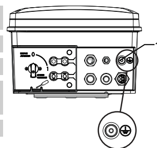
Kuva 25: Lisämaadoituspiste
