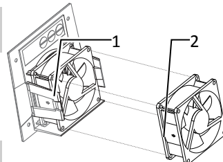
Kuva 28: Irrota tuulettimen liitin
