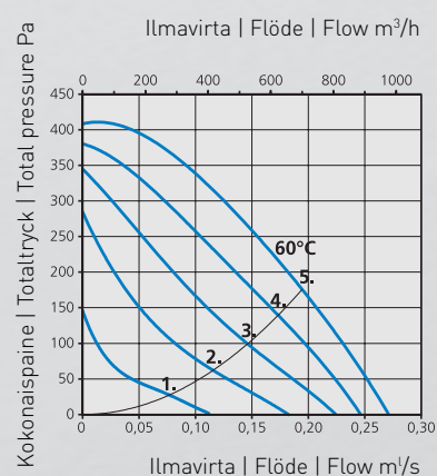
CK 250 A
